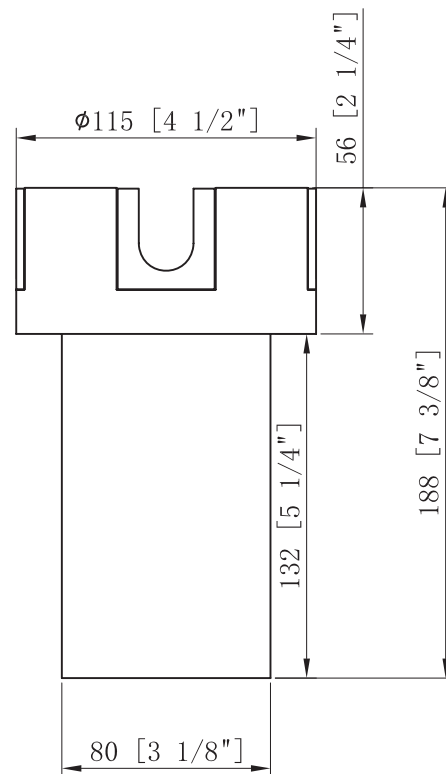
Conduit Mount
